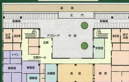
1階平面図
